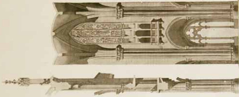
SECCION VERTICAL
